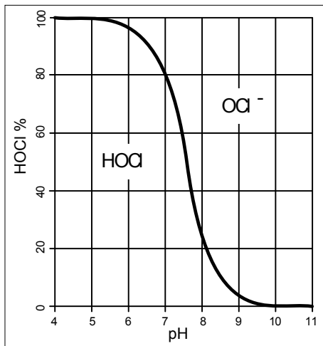
Fig. 36: HOCl/OCl - equilibrium
