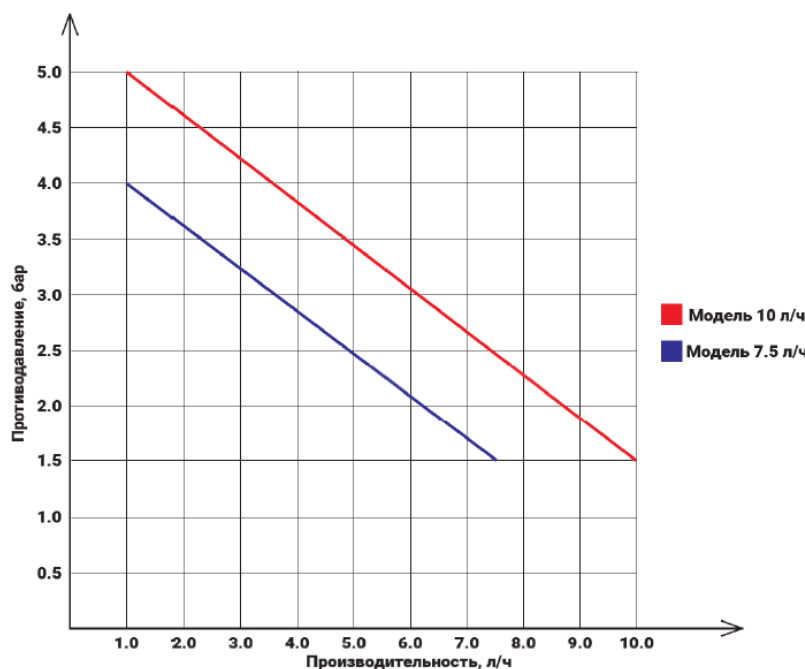
Рис.3 - График производительности мембранных насосов
