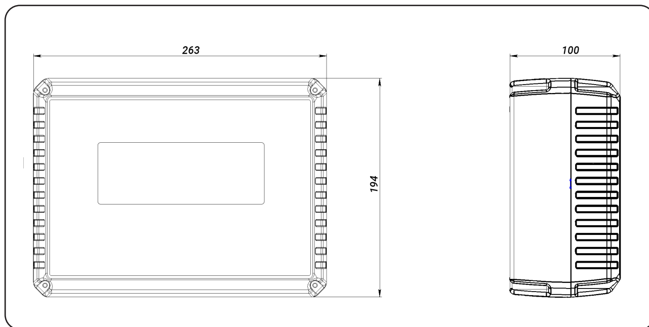
Рис.1 - Общие размеры Установки
