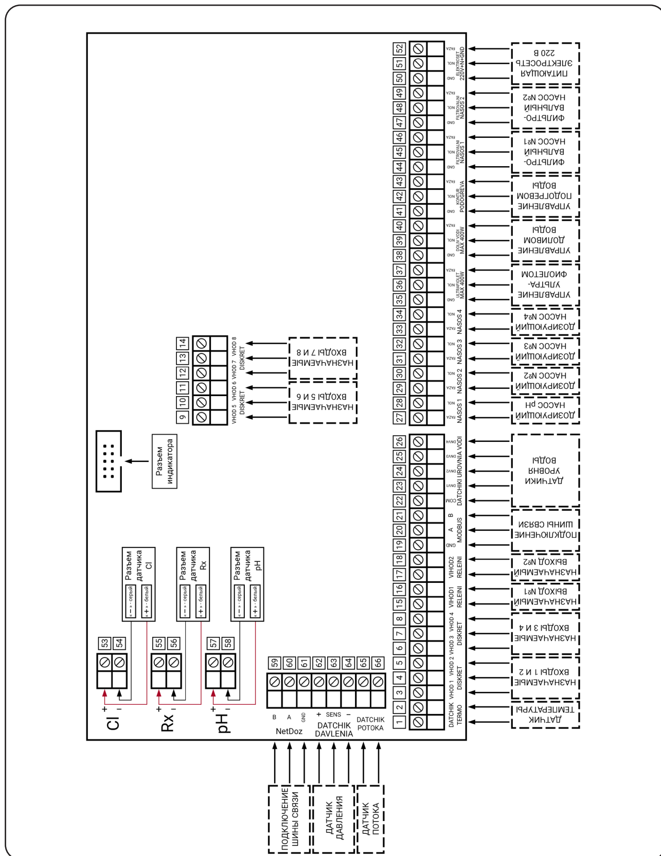
Рис.5 - Электрические подключения DOMINATOR-M PRO
