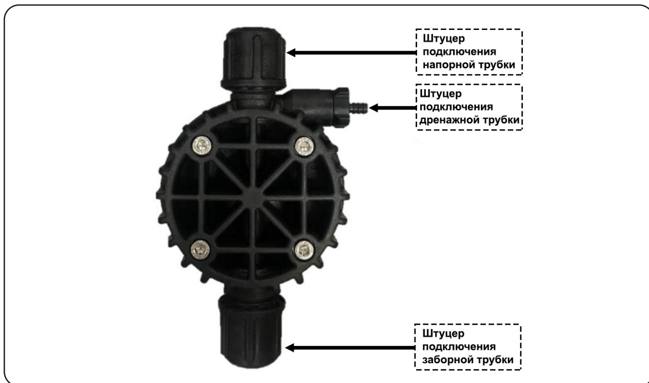
Рис.4 - Схема подключения трубок к мембранному насосу
