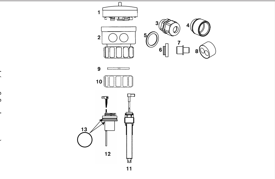
Fig. 5.1 Pièces de rechange, régulateur 8205 compact
