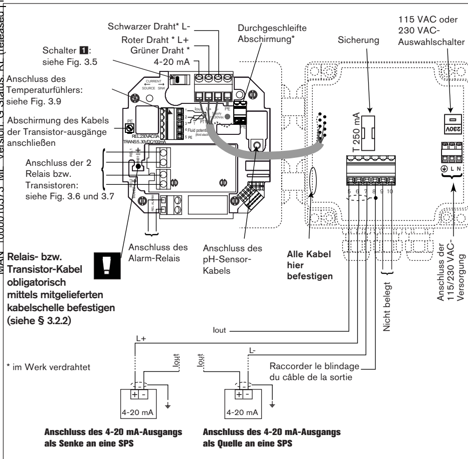
Fig. 3.10 anschluss Regler 8205, Wandmontage-Ausführung, 115-230 VAC
