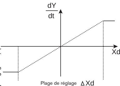
Fonction caractéristique
