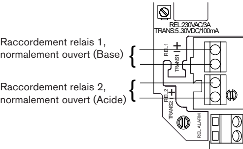
Version avec 2 relais
