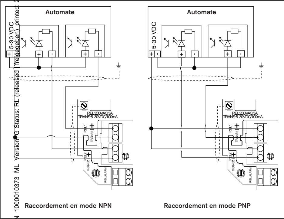
Fig. 3.7 Raccordement des sorties transistor à un automate
