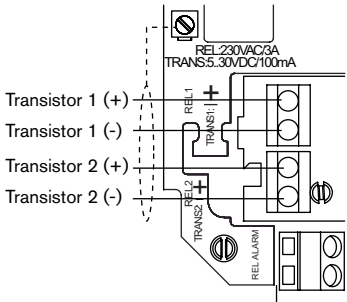
Version avec 2 transistors
