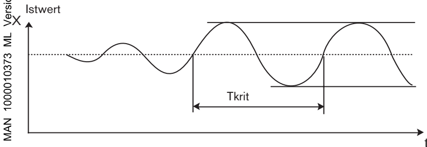
Bild : Verlauf der Regelgröße an der Stabilitätsgrenze
