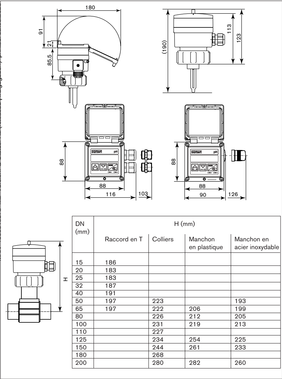
Fig. 2.3 Dimensions du régulateur de pH 8205 compact
