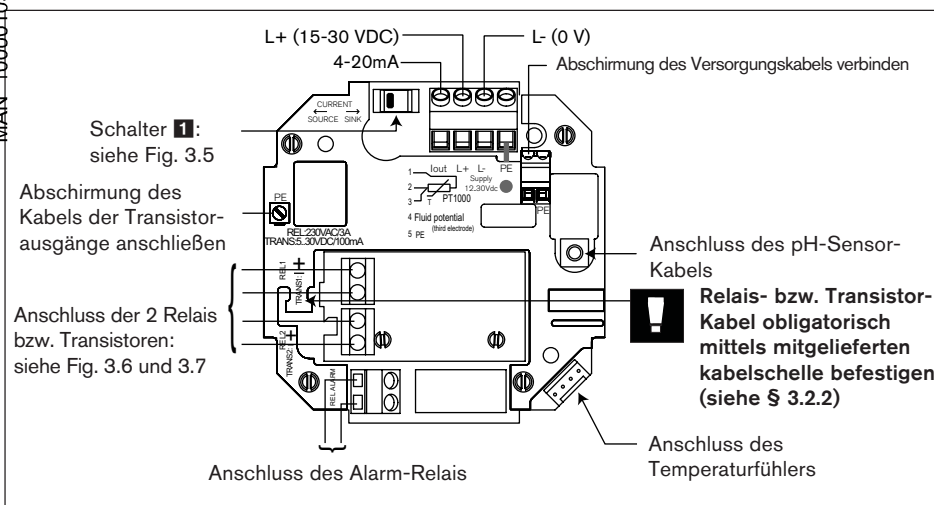
Fig. 3.4 Anschluss Kompakt-Regler 8205
