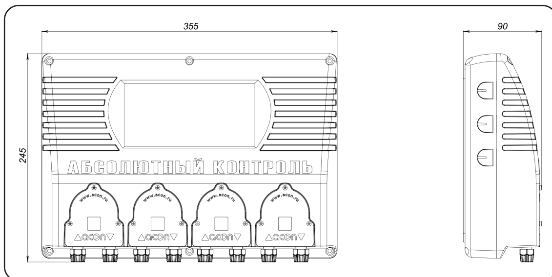
Рис.1 - Общие размеры Установки
