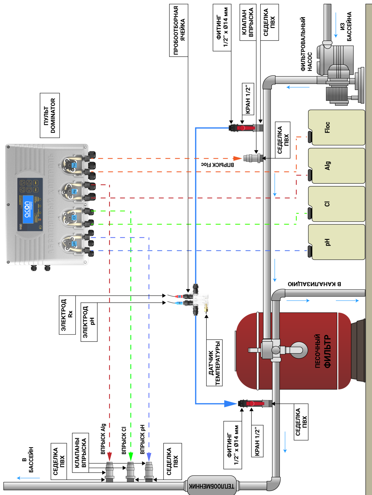
Рис.2 - Гидравлическая схема подключения DOMINATOR
