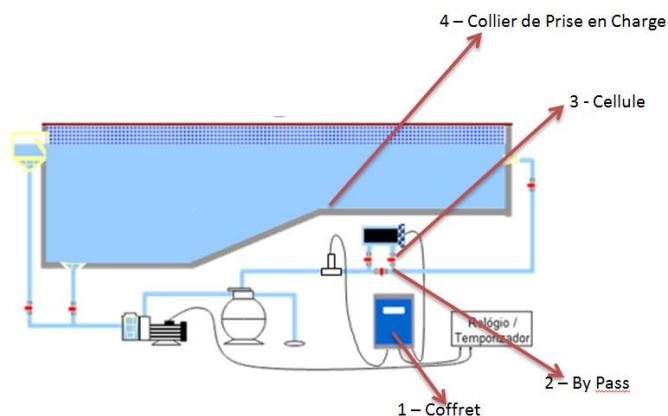
Fig 1- Système hydraulique
