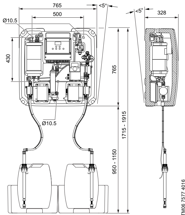
Fig. 19 Dimensions of OCD-162-5, -10
