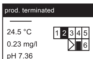
Fig. 33 Initial display
