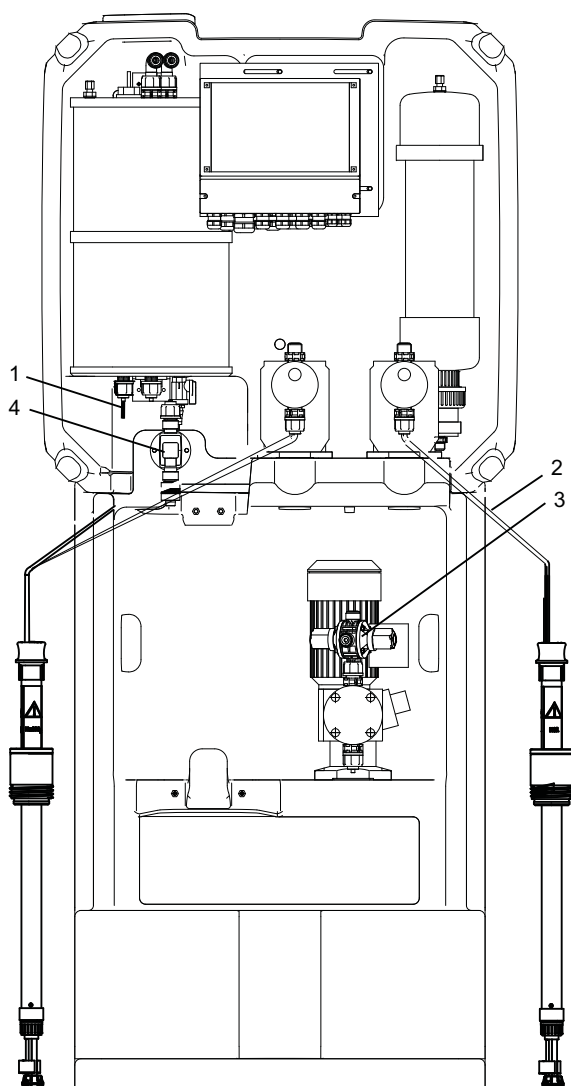
Fig. 24 OCD-162-30
