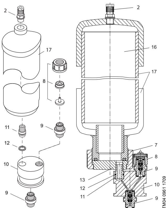
Fig. 47 OCD-162-30, -60
