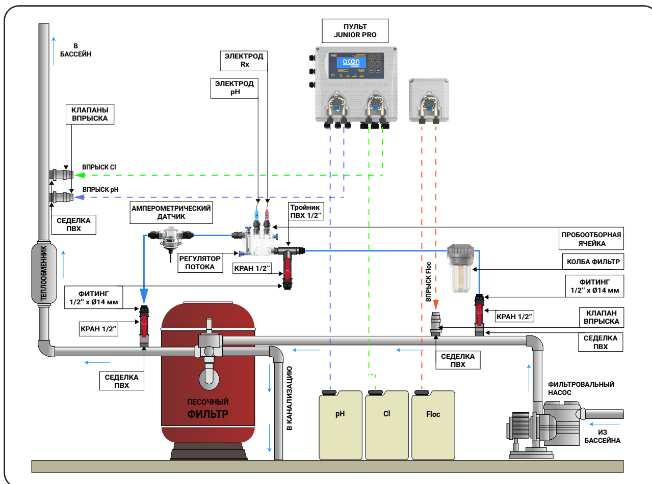
Рисунок 2 - Гидравлическая схема подключения JUNIOR PRO
