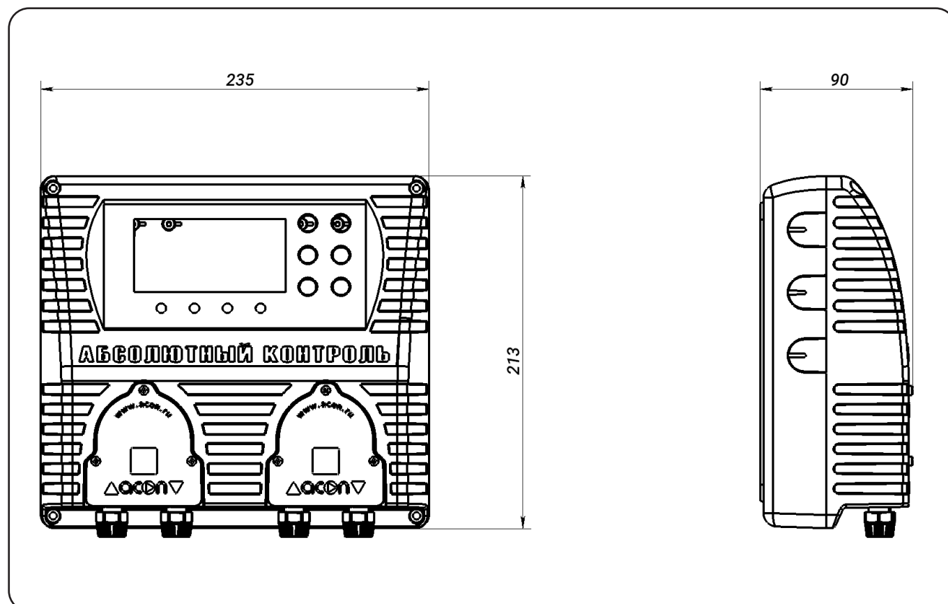
Рис. 1 - Общие размеры Установки
