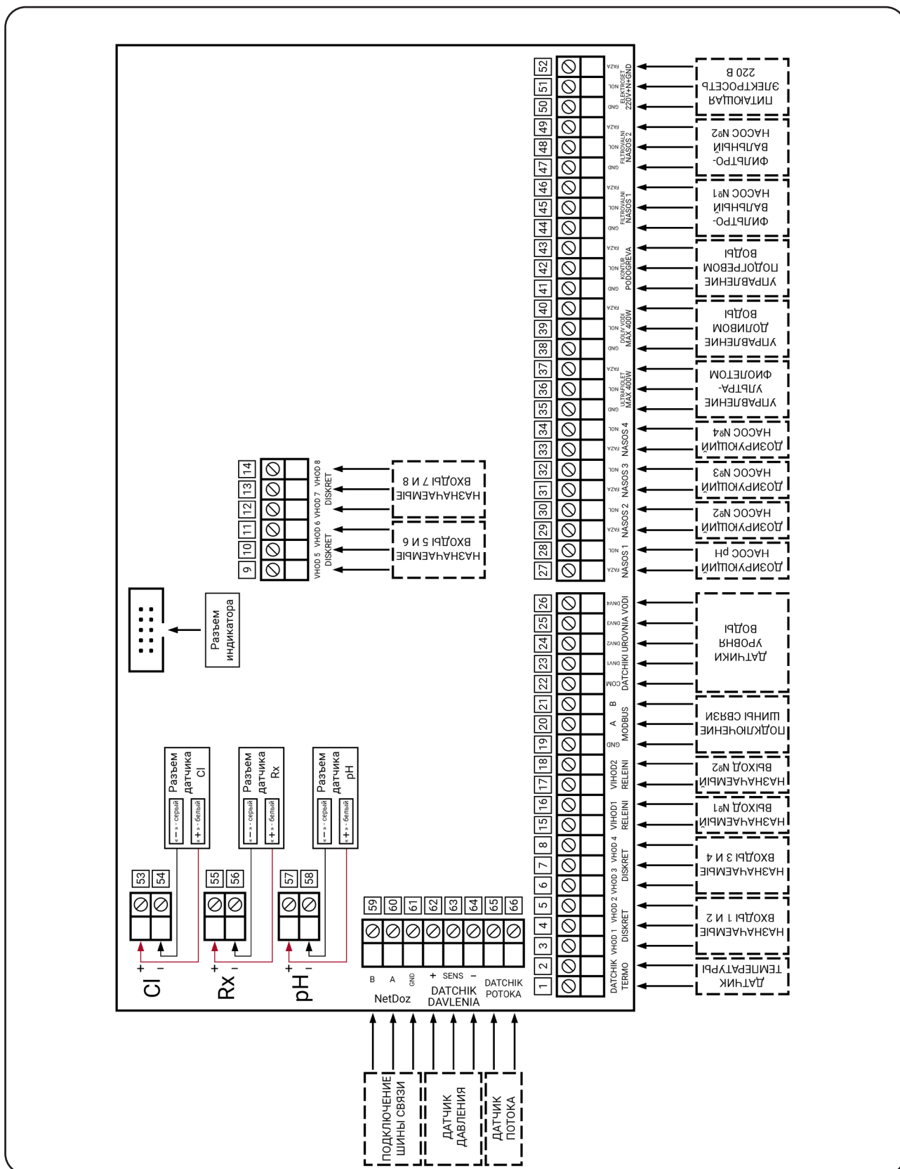
Рис.3 - Электрические подключения DOMINATOR PRO
