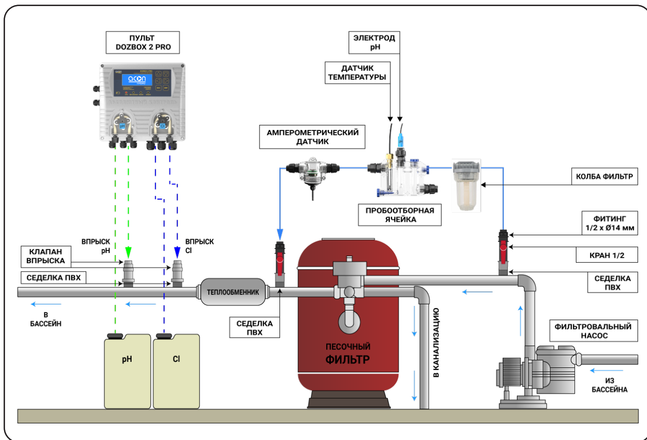
Рис.2 - Гидравлическая схема подключения DOZBOX 2 PRO
