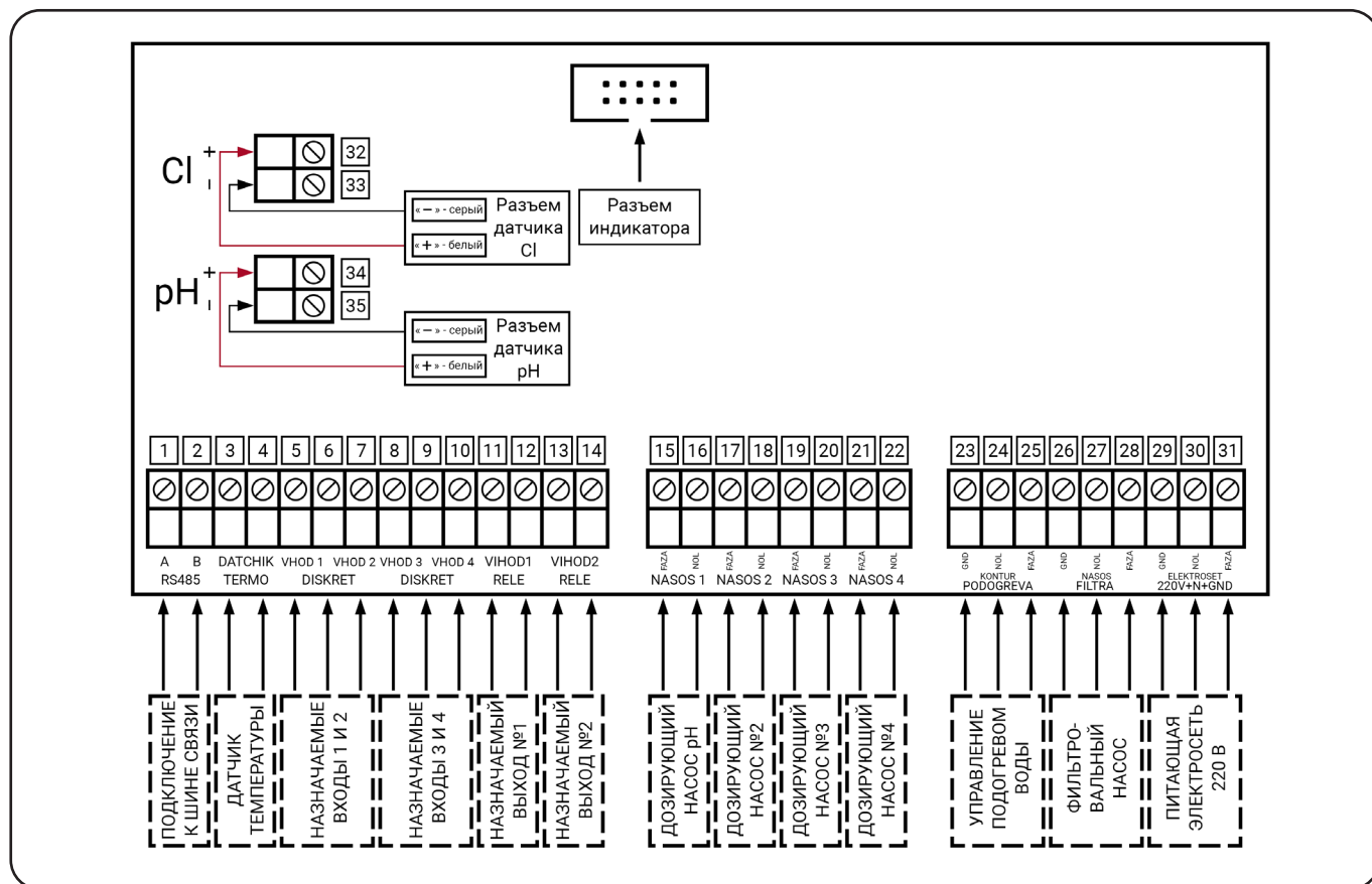
Рис.3 - Электрические подключения DOZBOX 2 PRO
