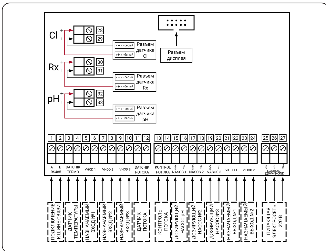
Рисунок 4 - Электрические подключения JUNIOR-M PRO
