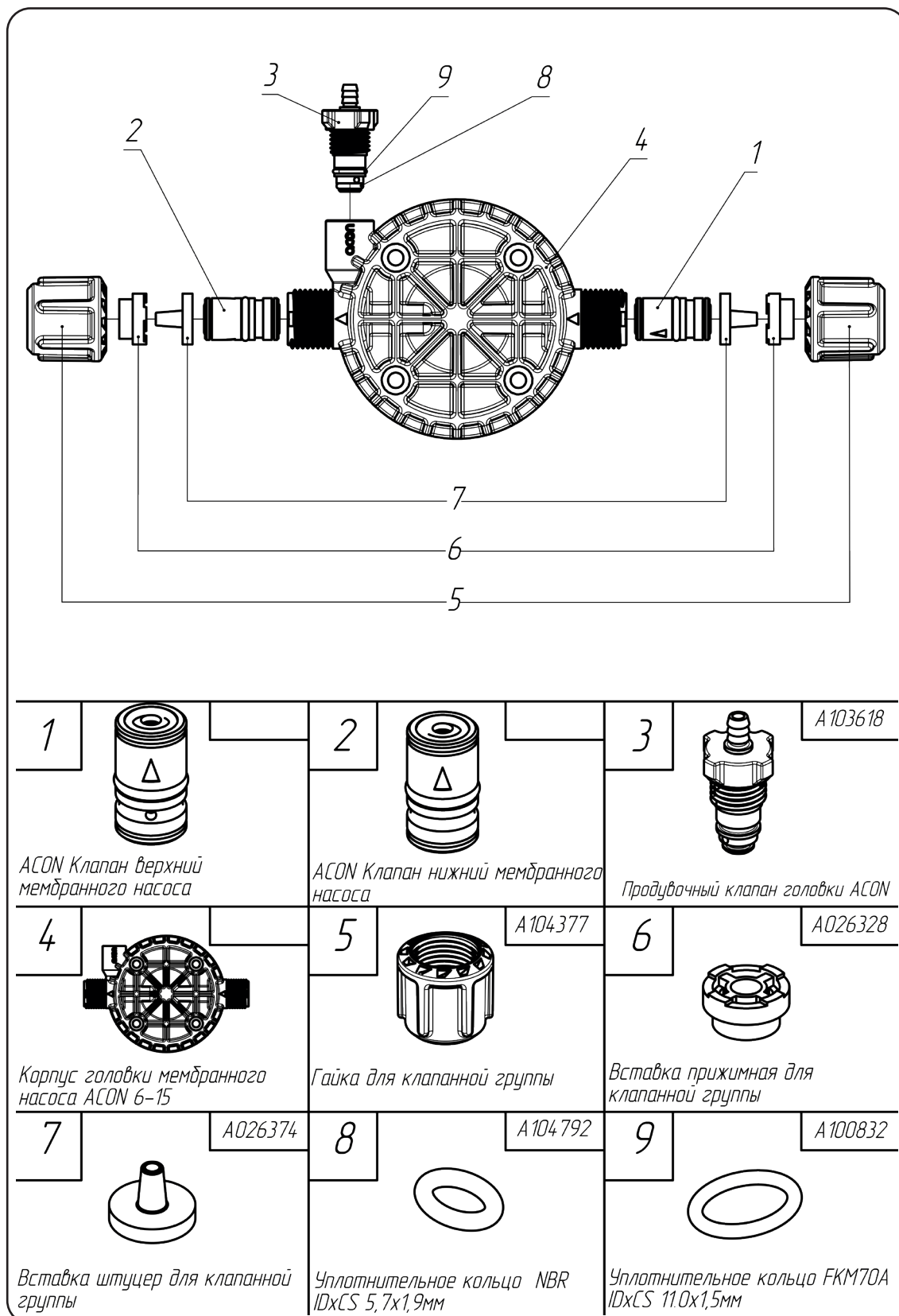
Рисунок 6. Основные детали головки мембранного насоса
