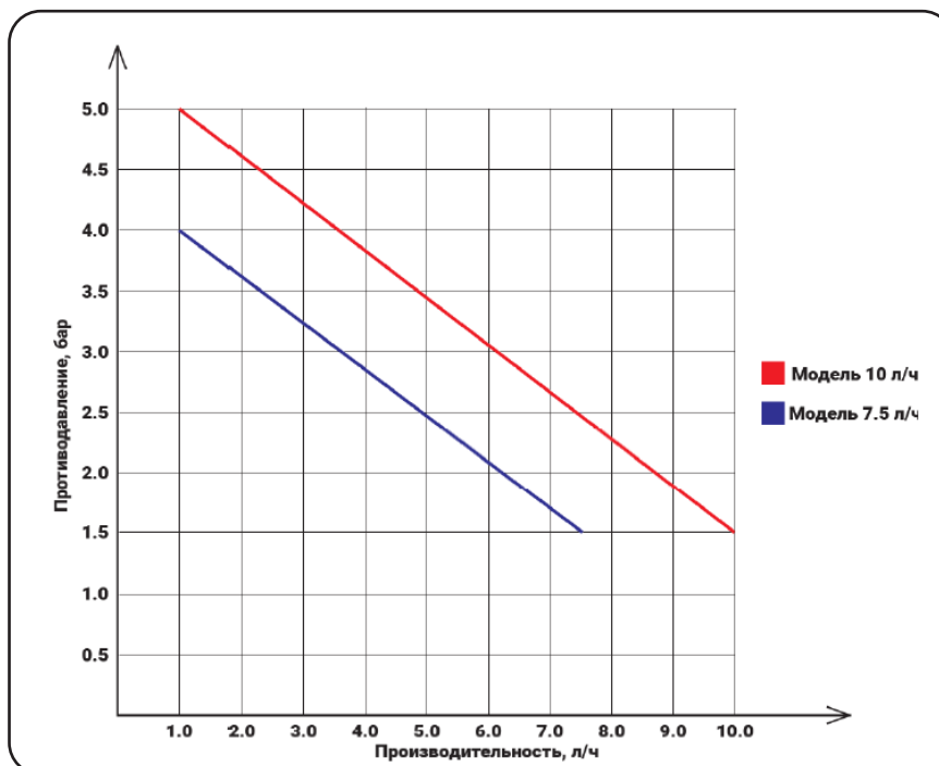
Рисунок 3 - График производительности мембранных насосов
