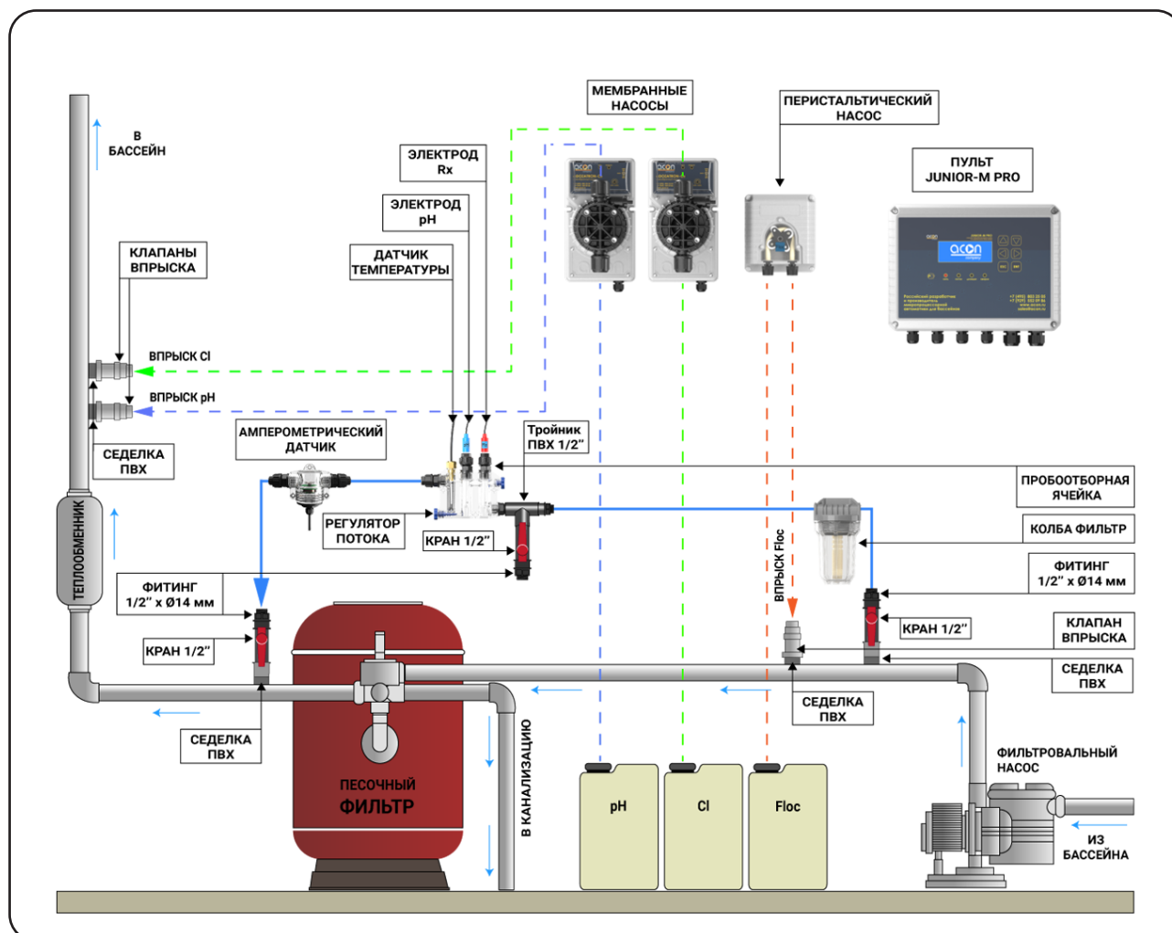
Рисунок 2 - Гидравлическая схема подключения JUNIOR-M PRO
