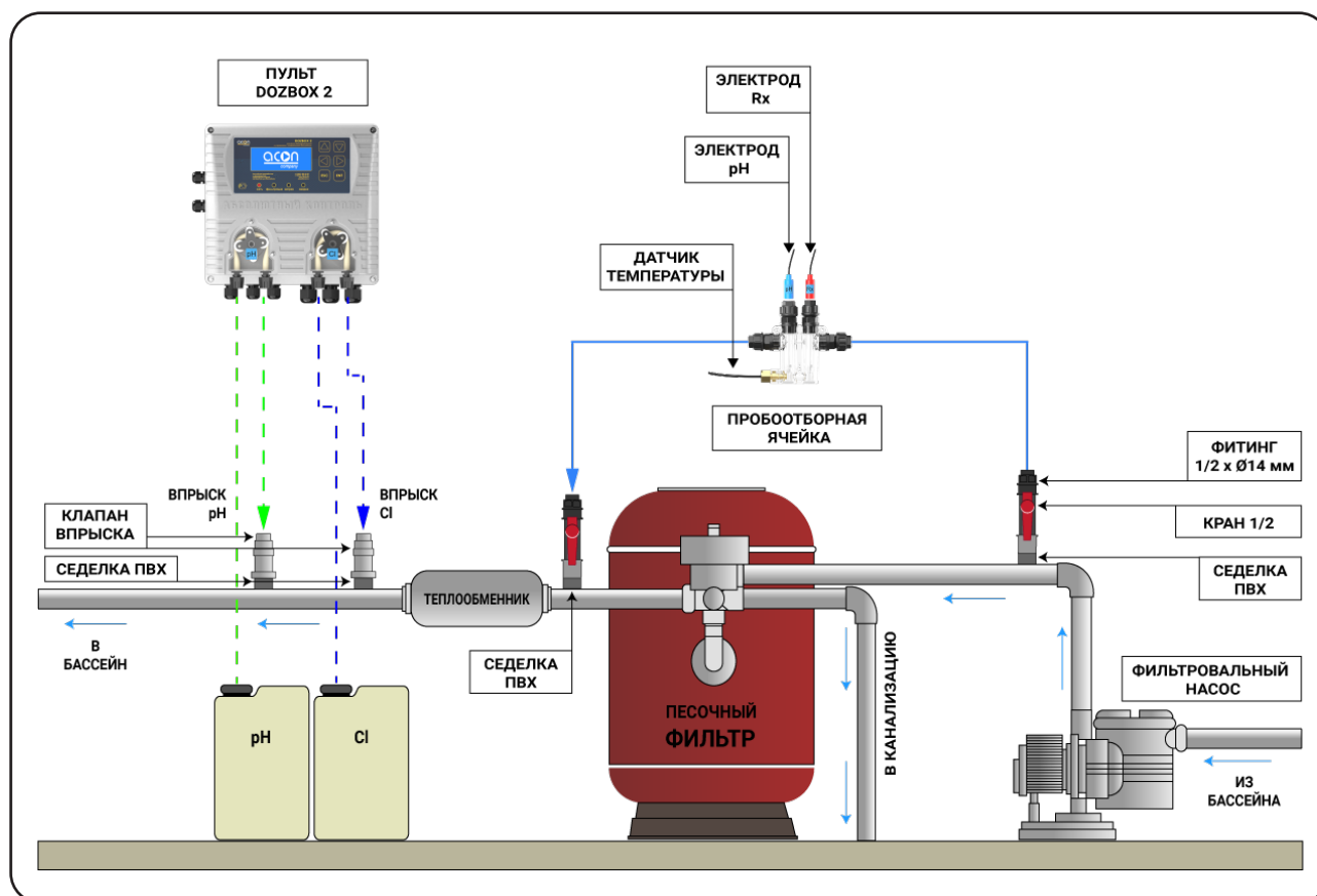
Рис.2 - Гидравлическая схема подключения DOZBOX 2
