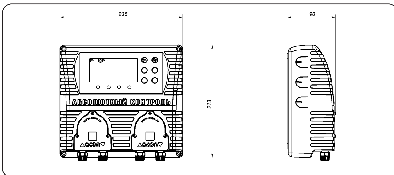
Рис.1 - Общие размеры Установки
