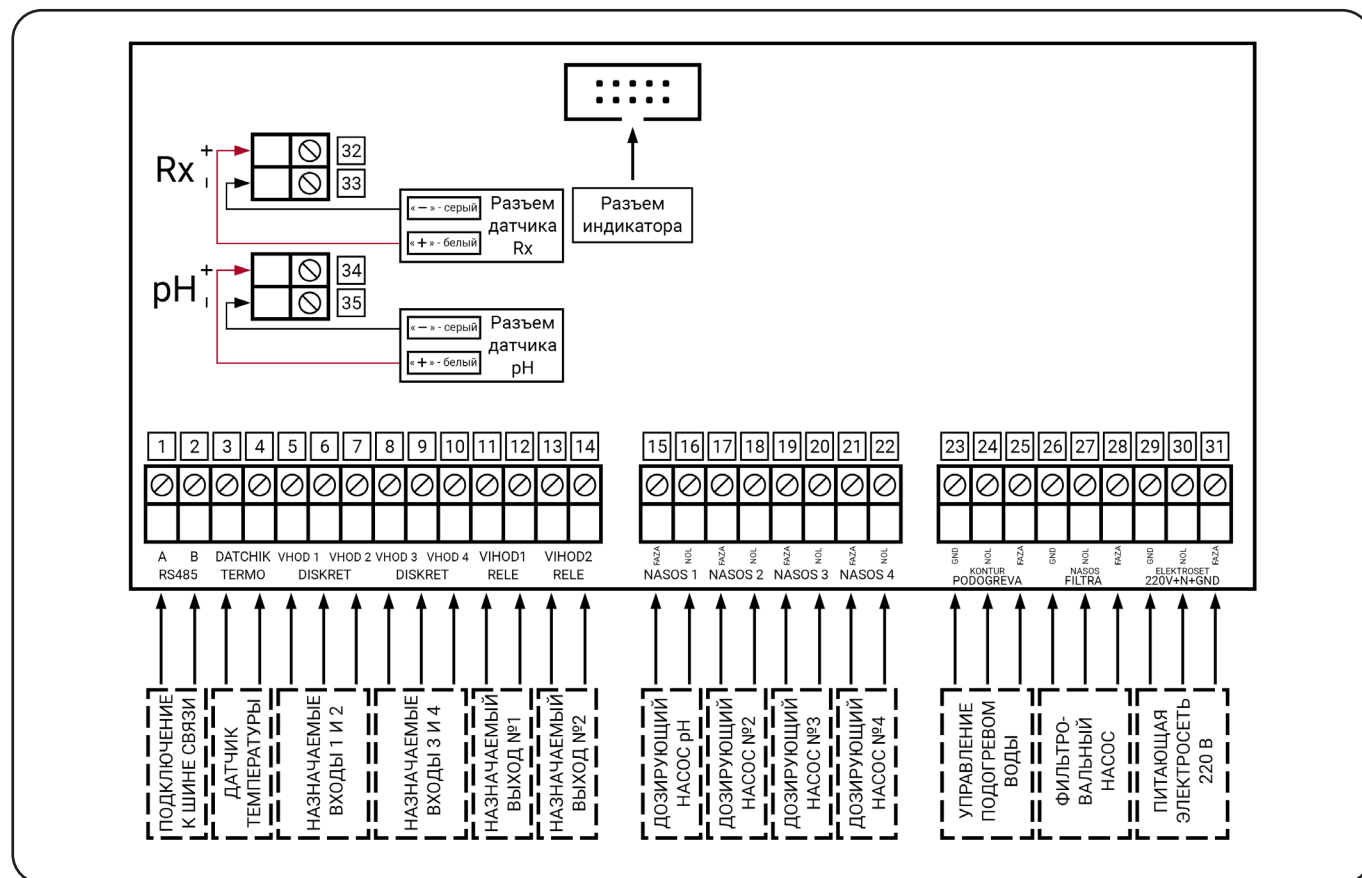
Рис.3 - Электрические подключения DOZBOX 2
